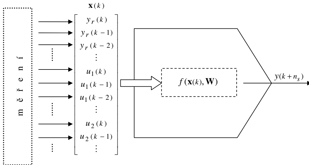
Obr. 5: Obecné schéma komplikovaného statického modelu s vektorem měřených vstupních veličin u a historií měřené (reálné) výstupní (modelované) veličiny y_r , x označuje vstupní vektor do modelu.
