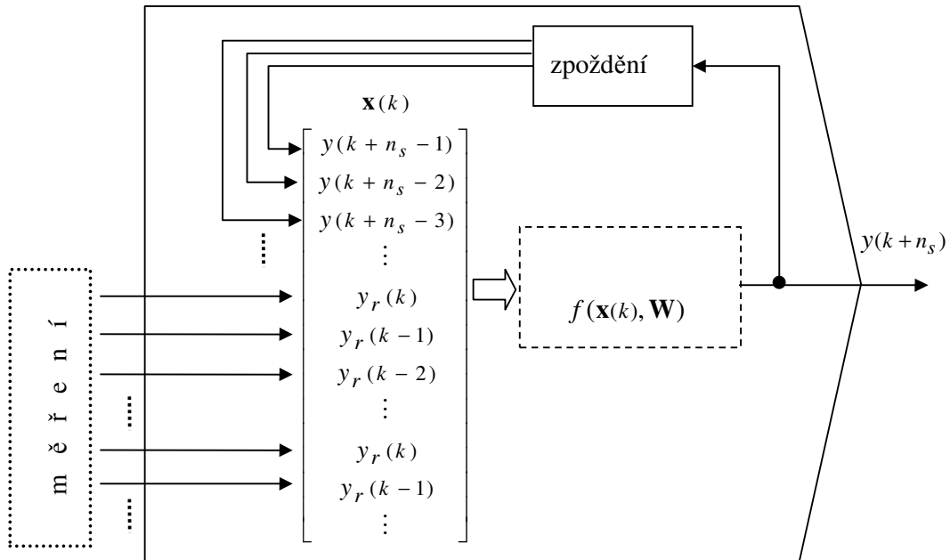
Obr. 4: Reálnější příklad dynamického prediktivního modelu s měřenou modelovanou veličinou y_r a zpětnými vazbami s výstupní (modelovanou) veličinou y (pro model je měřením dostupná jediná veličina a to jen ta modelovaná).
