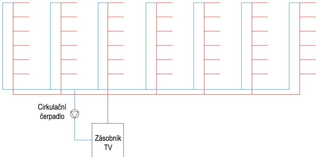
Obr. 1 Základní schéma rozvodu TV s cirkulací
