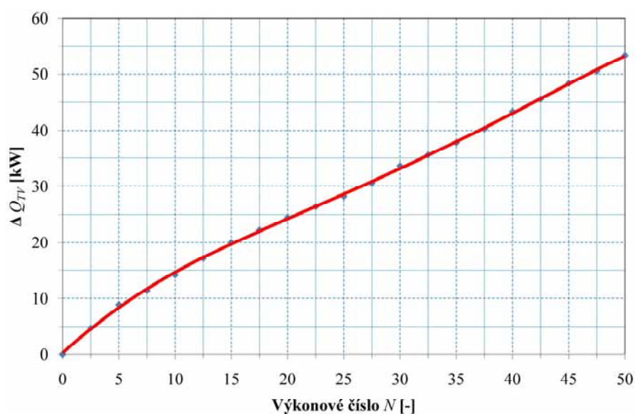
Obr. 1 Zvýšený výkon kotle k ohřevu teplé vody podle koeficientu potřebu zásobníku TV N
